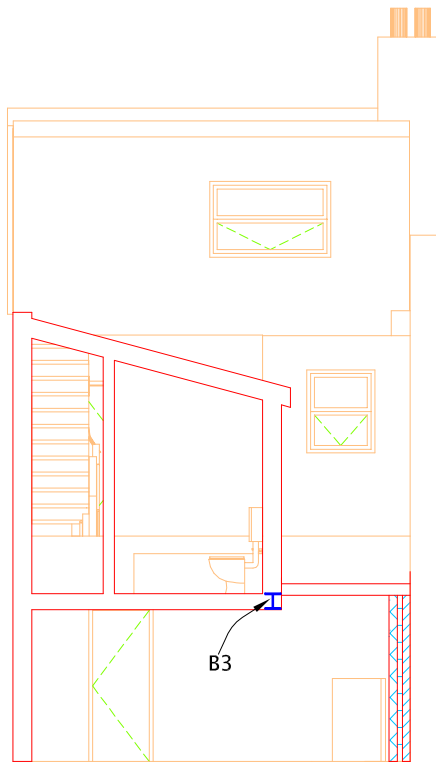
Section D-D
